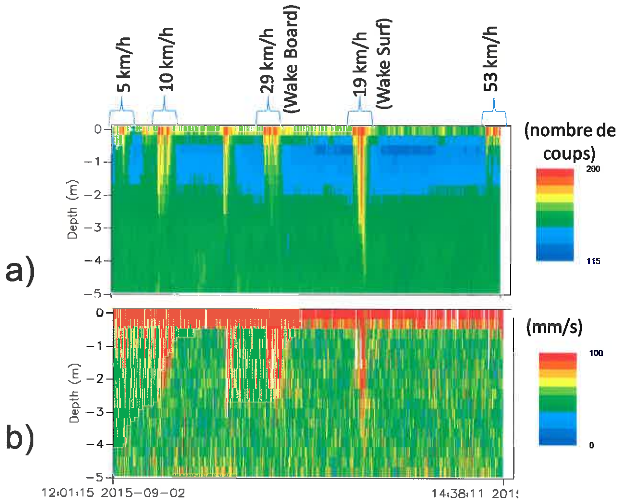
Figure 7: Intensité moyenne (a) et vitesse générées (b) lors du passage des « Wake Boat » à différentes vitesses pour le 1 er jour d'essai
