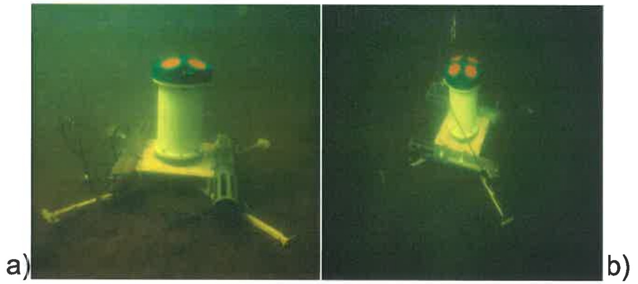
Figure 11 : Vue du dispositif expérimental avant (a) et 2 minutes après (b) le passage d'un « Wake Boat »
