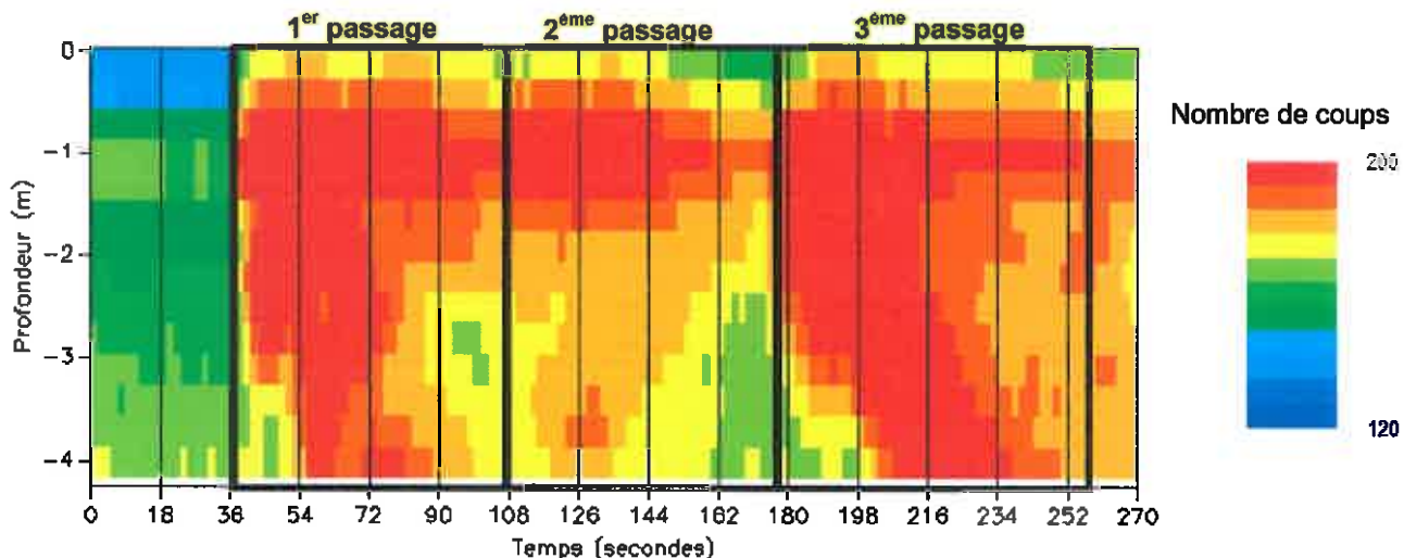
Figure 9: Zoom de la figure 8a sur les passages de bateaux en mode « Wake surf » pour le 2 ème jour sur le Lac des Sables
