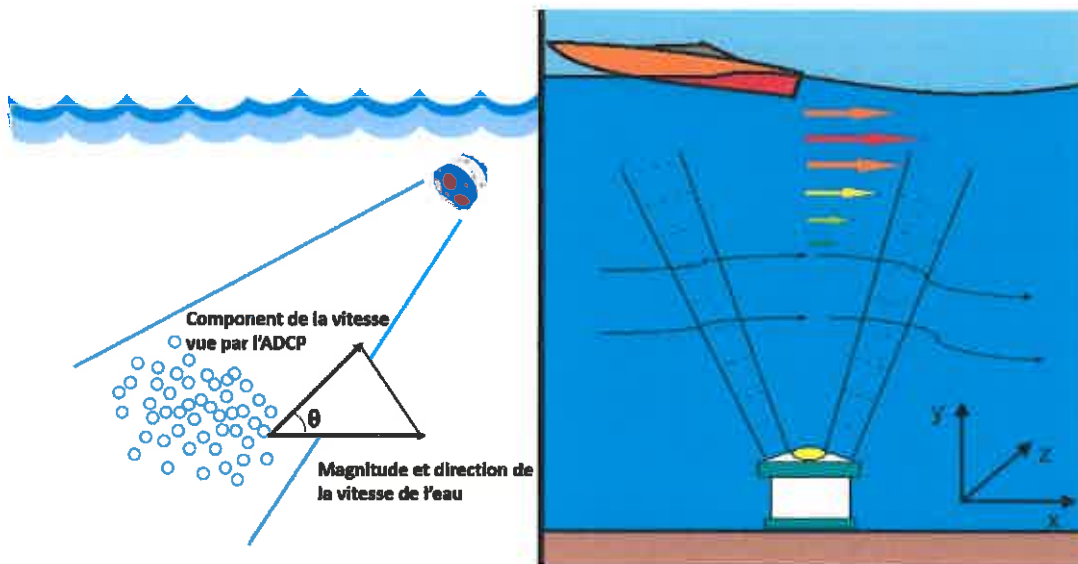
Figure 5: Mesures de courant en 3 dimensions (RD Instrument, 1989)
